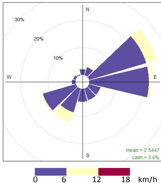
Figura 3: Porcentaje de frecuencias por dirección predominante para febrero 2024. Leyenda de colores indica la velocidad en km/h.
